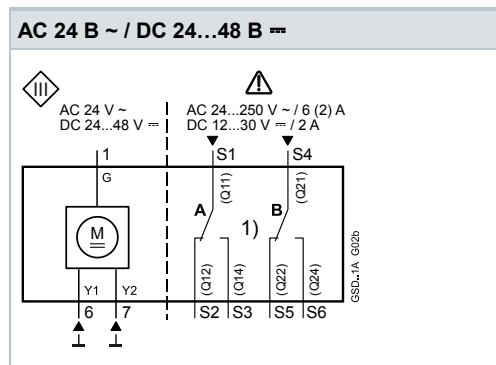
GSD14..1A (Открыть-закрыть, 3-точечный)
