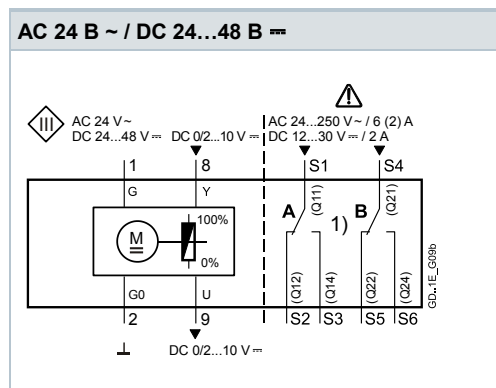
GSD16..1A (Плавное регулирование)
